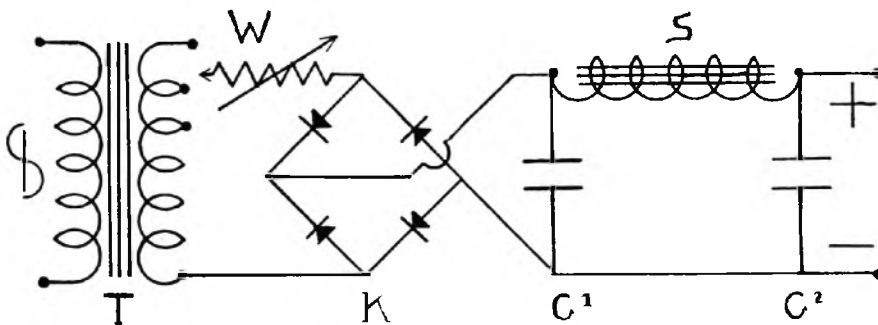
Principe-schema Gloeistroom-apparaat
